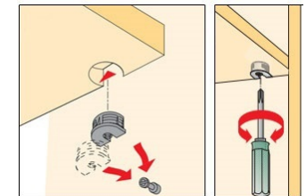
Схема установки стяжки рафикс Ф-1
