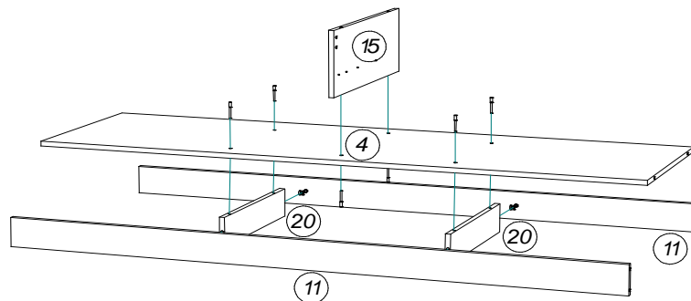
Схема сборки цокольной коробки (рис.4)
