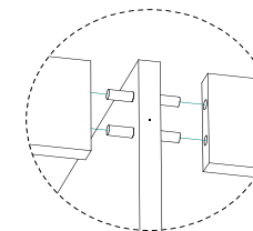
Схема установки шкантов 8x50 (рис.9)
