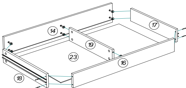
Схема сборки ящика (рис.3)
