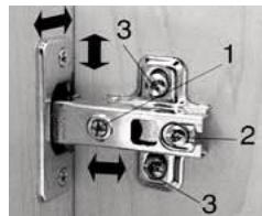
Схема регулировки четырехшарнирной петли (рис.14)
