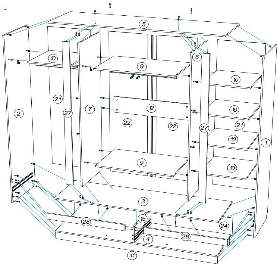
Схема сборки шкафа (рис.1)
