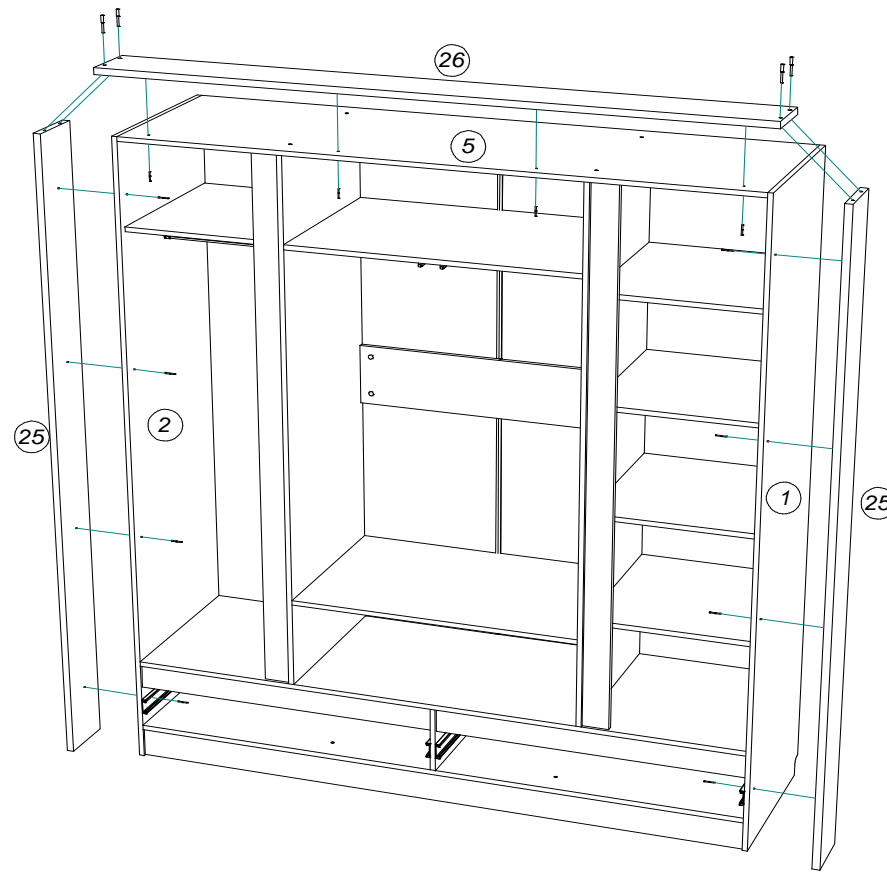
Схема установки обкладки (рис.2)
