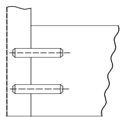
Схема установки шкантов 8x30 (рис.11)
