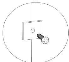
Схема установки скрепки для ДВП (рис.12)
