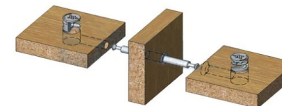
Схема установки эксцентриковой стяжки с двухсторонним штоком (рис.10)
